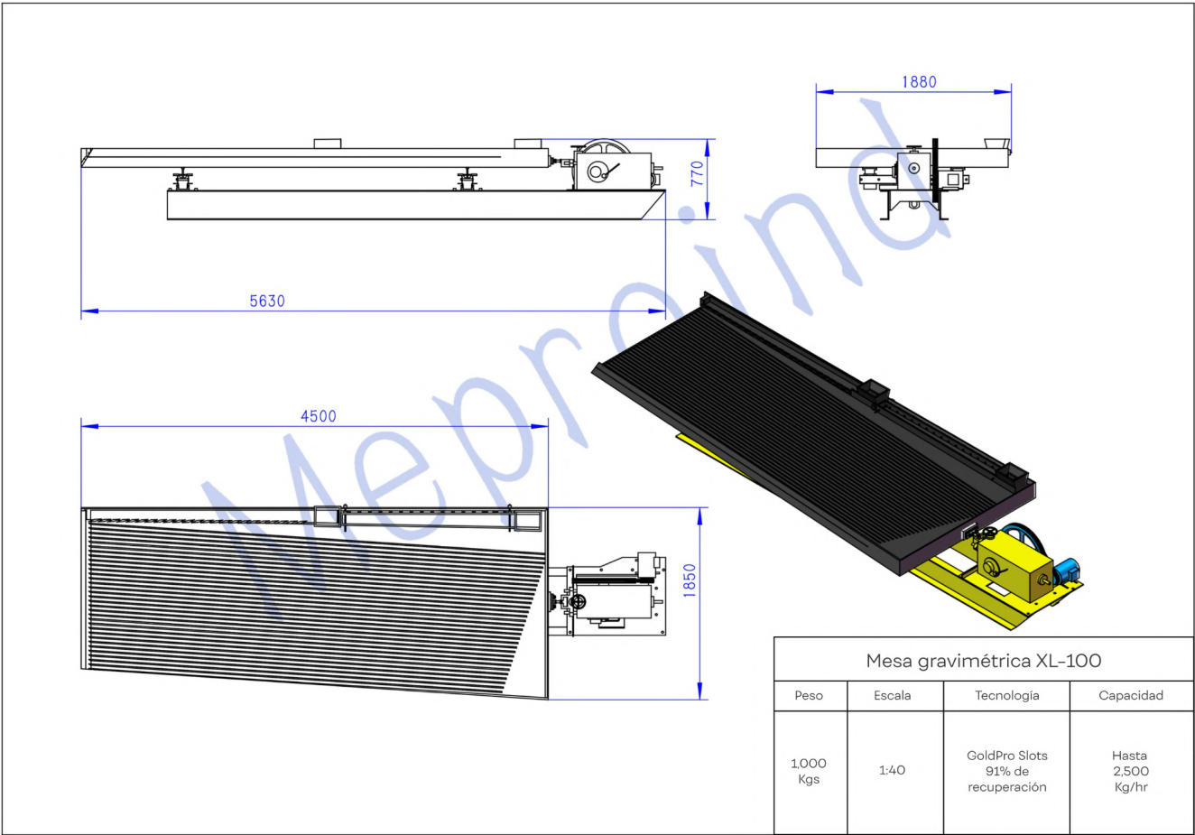
Imagen 1: Plano de la mesa gravimétrica XL-100 (2.5 ton/hr).
