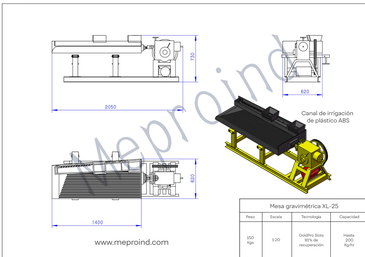
Imagen 2: Plano de la mesa gravimétrica XL-25 (200 kg/hr).
